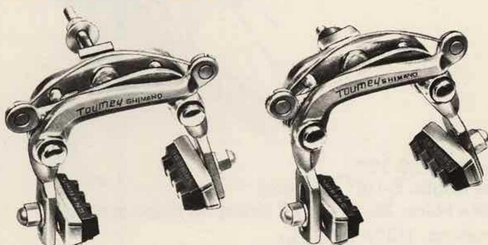
Center Pull Type CC-65 type Model.: B-110 CC-75 type Model.: B-120
