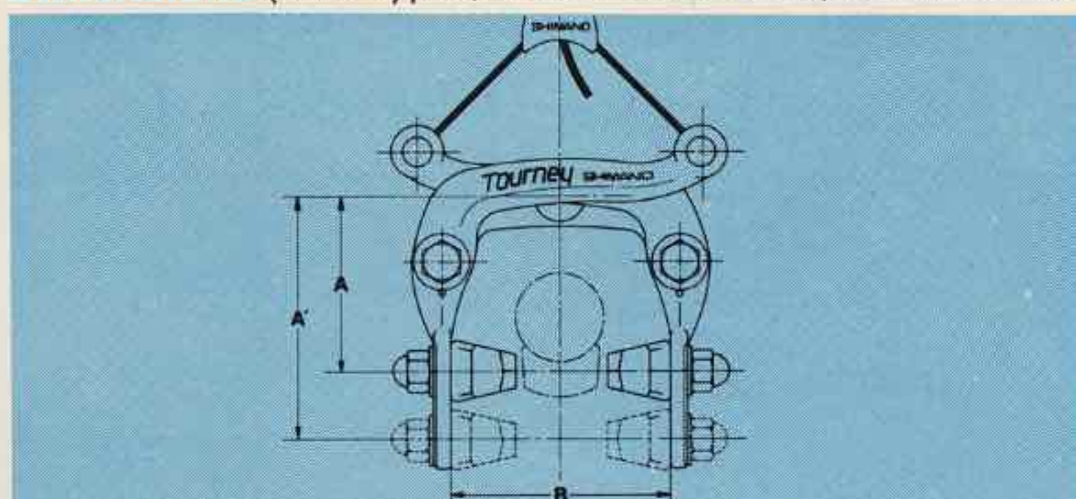
Center Pull Type CC-65 type Model.: B-110 CC-75 type Model.: B-120
